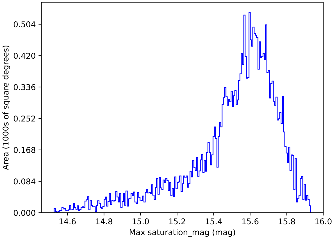
roman_v3.3_10yrs All sky i band: Max saturation_mag
