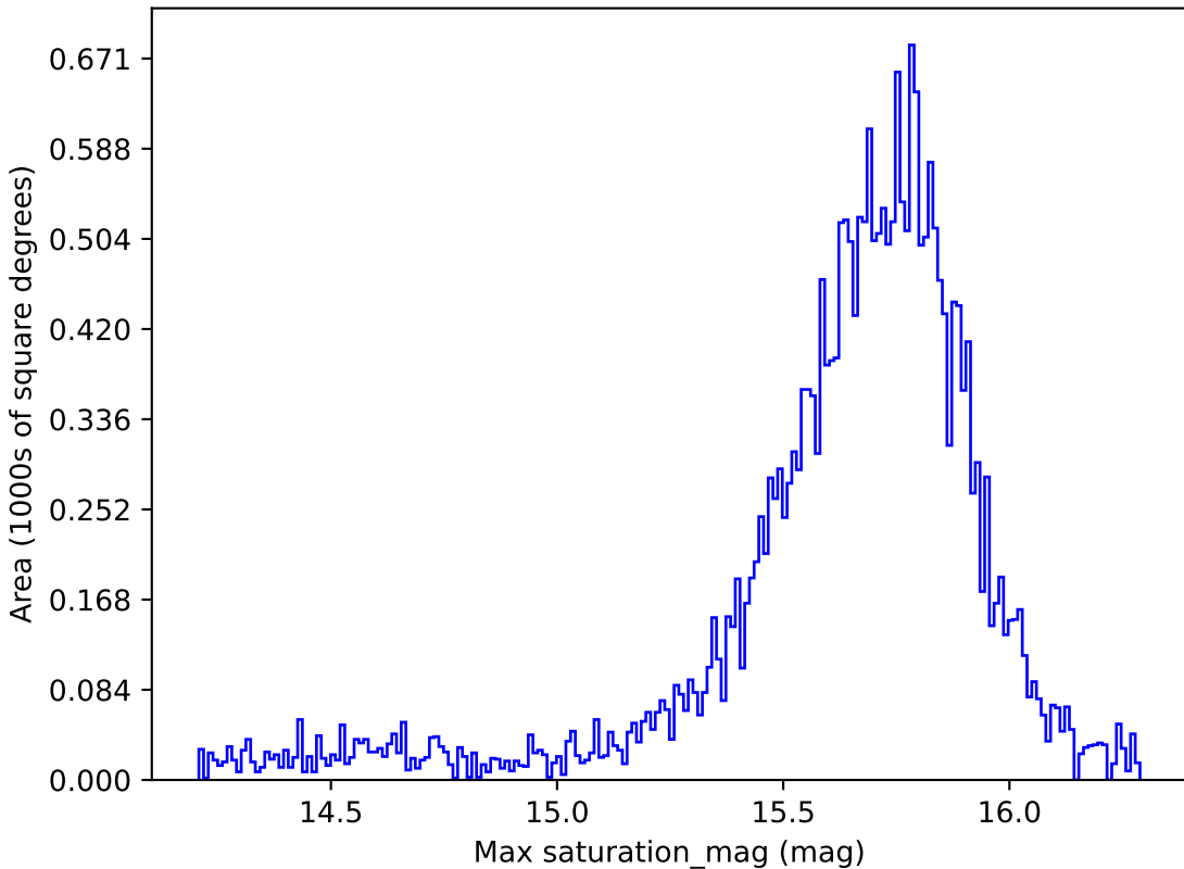
roman_v3.3_10yrs All sky g band: Max saturation_mag
