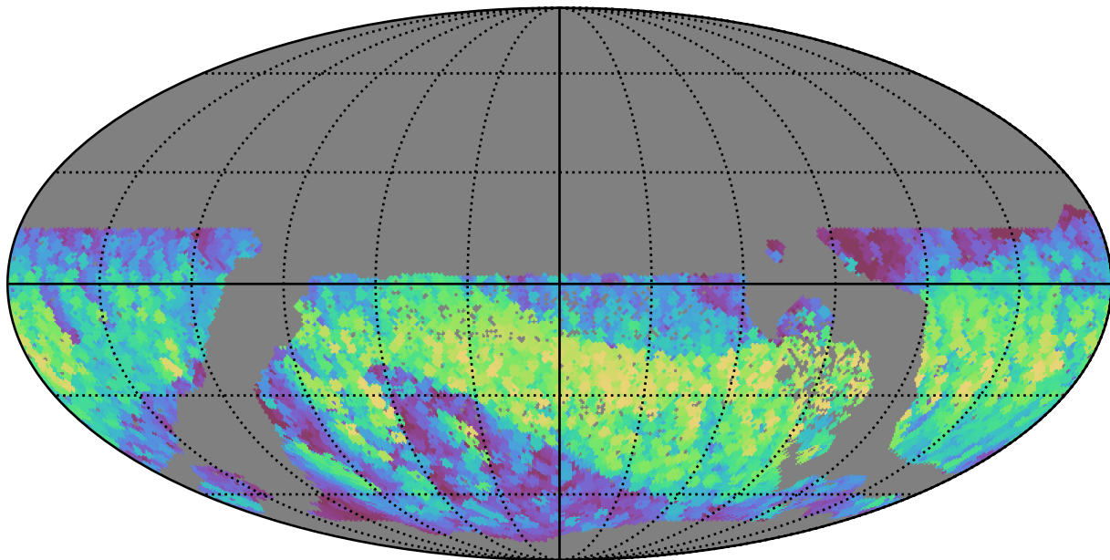
roman_v3.3_10yrs WFD z band: Max normairmass
