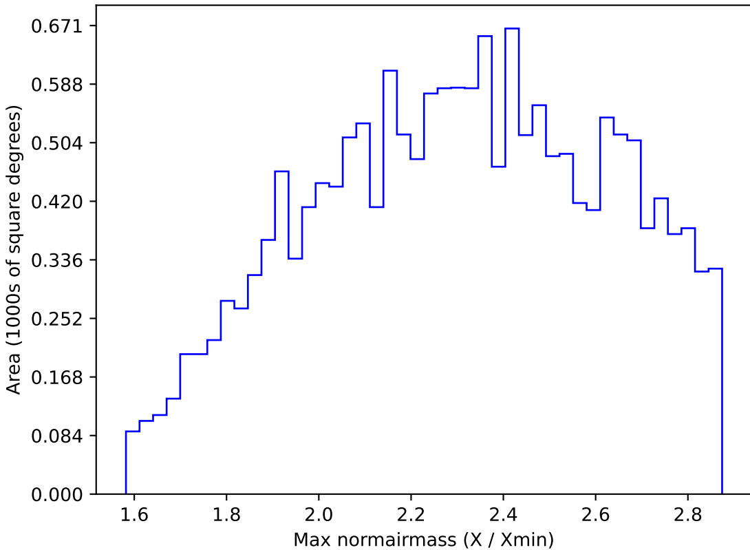
roman_v3.3_10yrs WFD z band: Max normairmass
