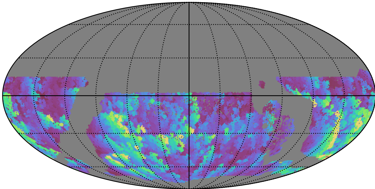
roman_v3.3_10yrs WFD u band: Max normairmass
