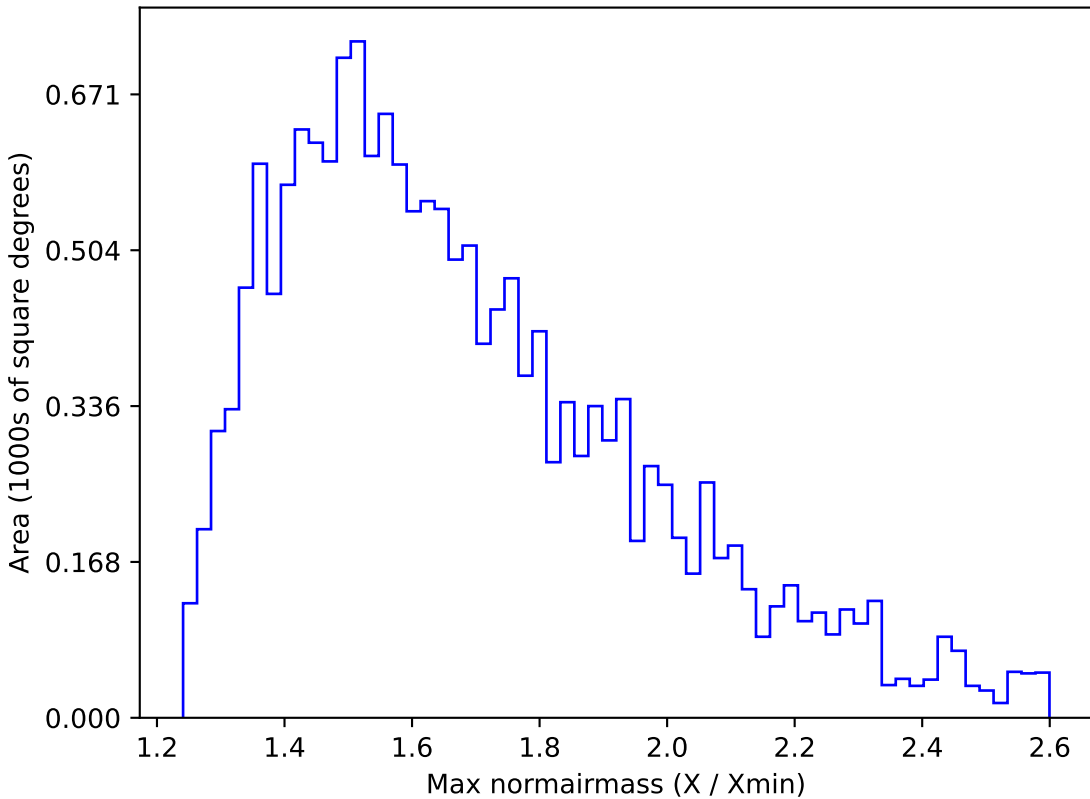
roman_v3.3_10yrs WFD u band: Max normairmass
