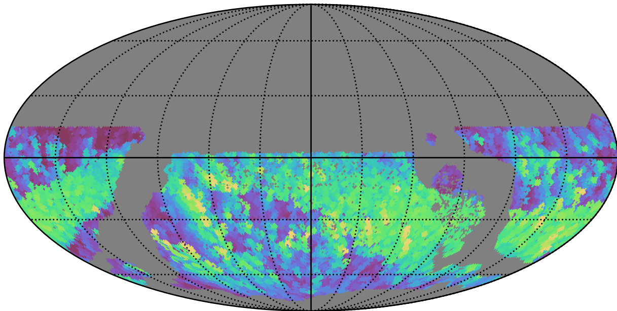
roman_v3.3_10yrs WFD r band: Max normairmass
