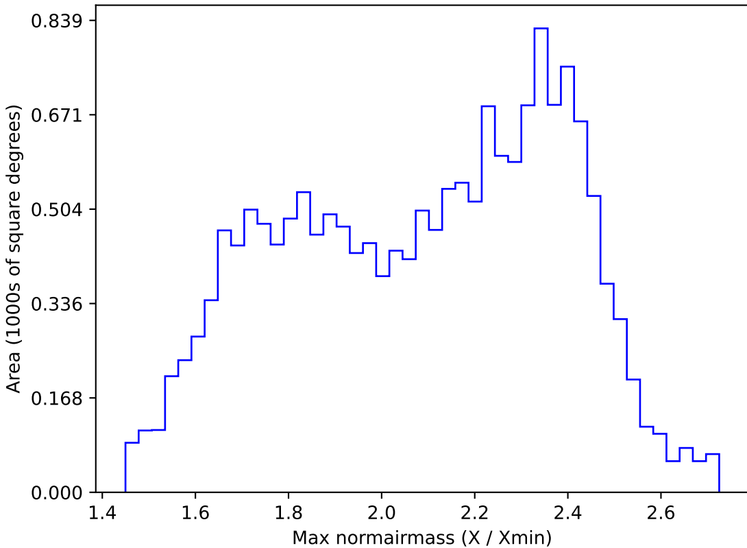
roman_v3.3_10yrs WFD r band: Max normairmass
