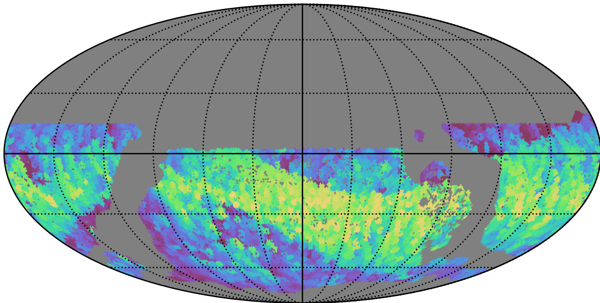
roman_v3.3_10yrs WFD i band: Max normairmass
