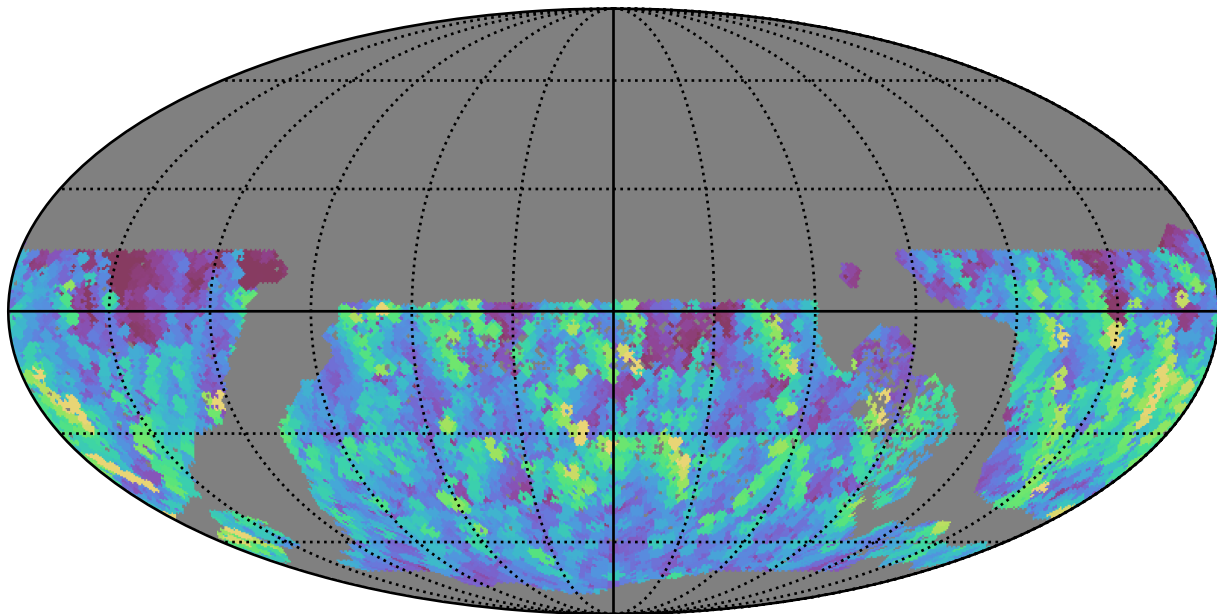
roman_v3.3_10yrs WFD g band: Max normairmass
