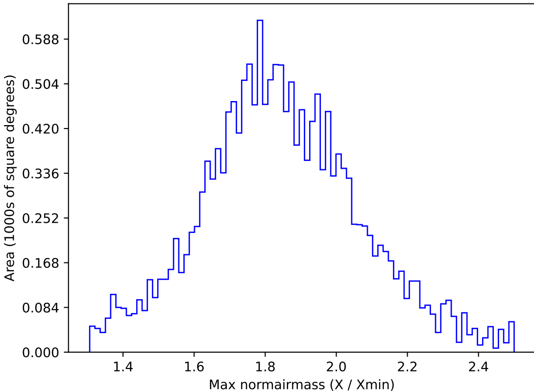
roman_v3.3_10yrs WFD g band: Max normairmass
