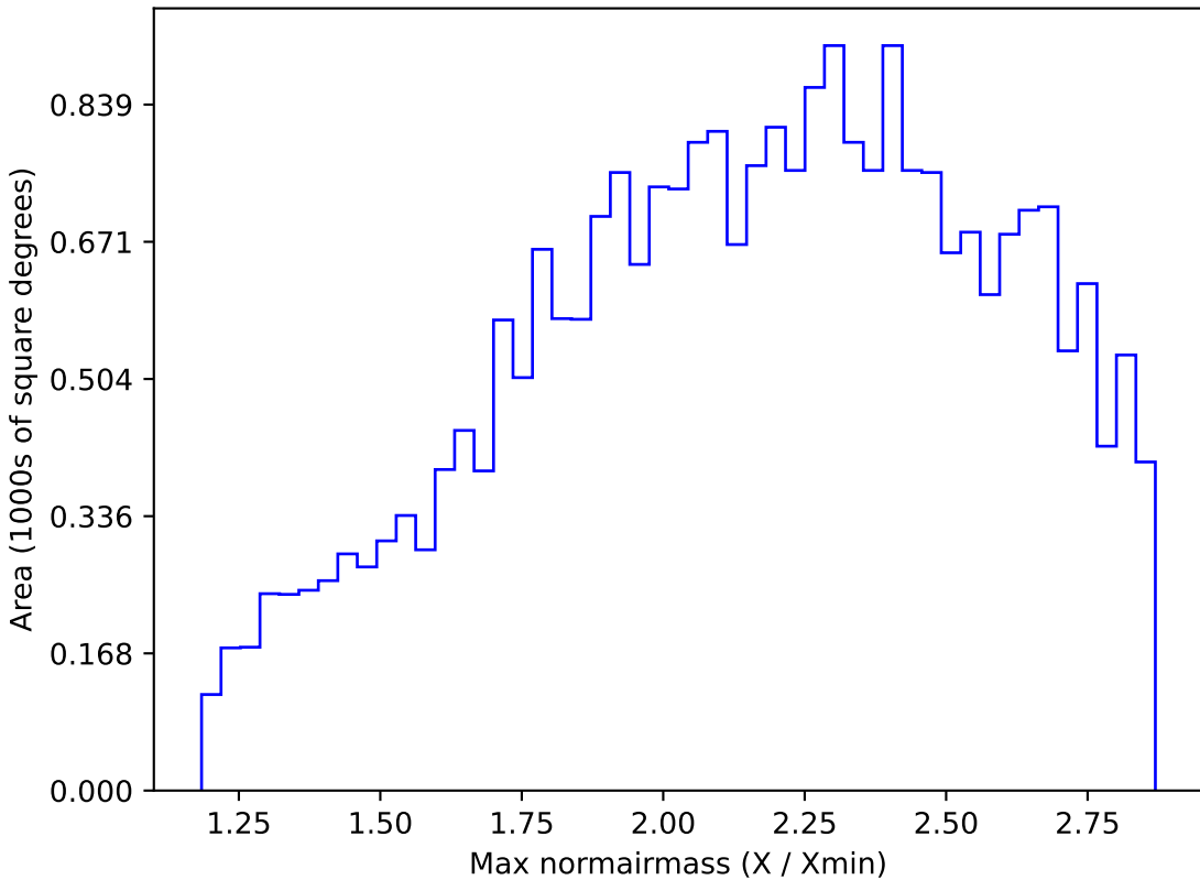
roman_v3.3_10yrs All sky z band: Max normairmass
