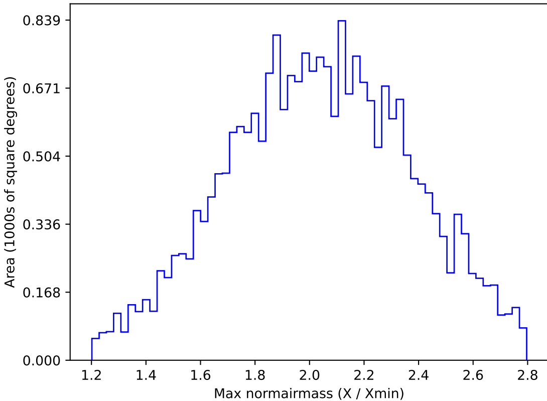
roman_v3.3_10yrs All sky y band: Max normairmass
