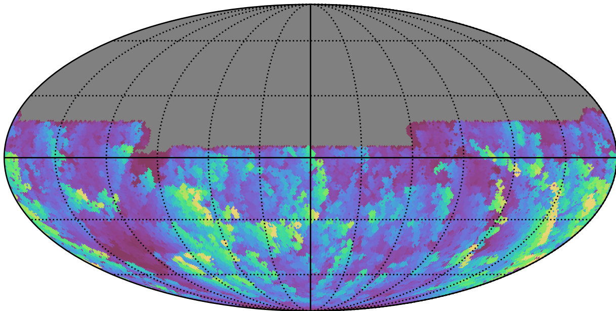
roman_v3.3_10yrs All sky u band: Max normairmass
