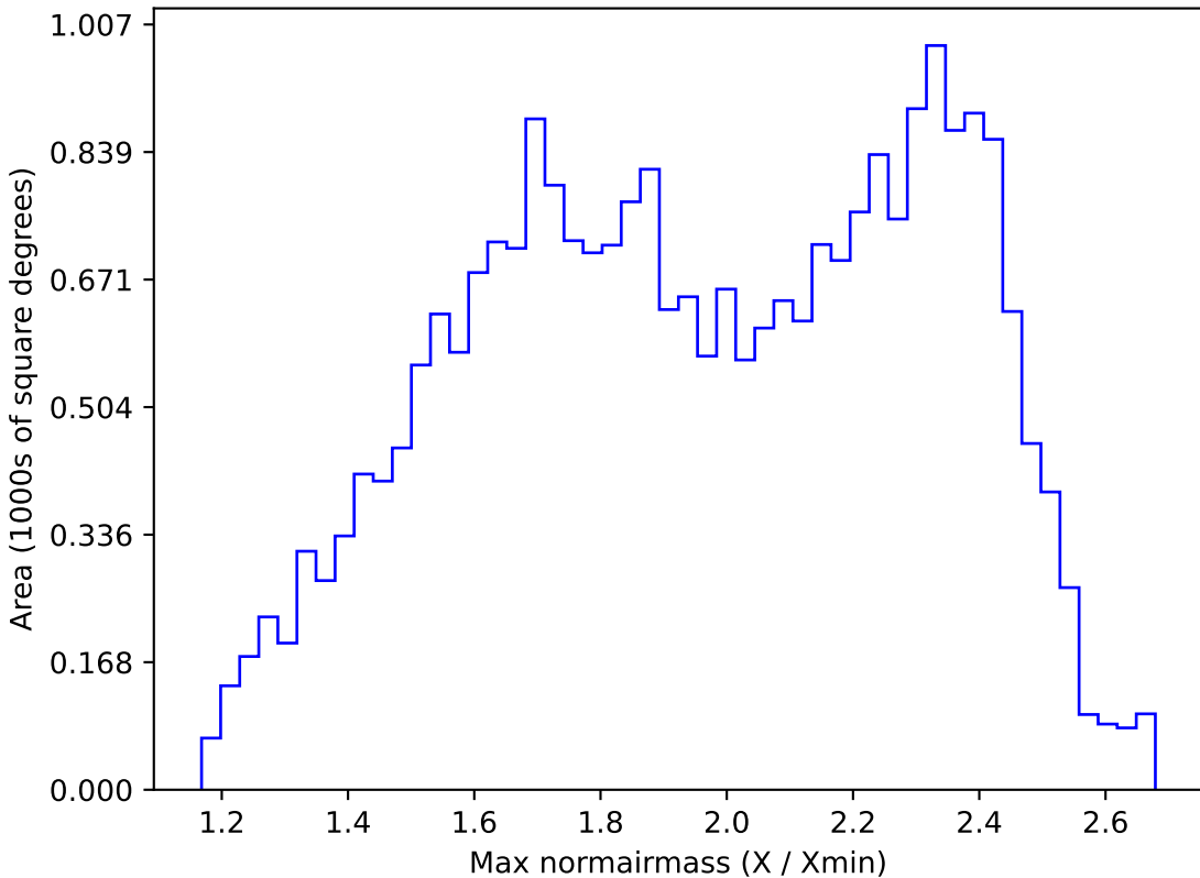
roman_v3.3_10yrs All sky r band: Max normairmass
