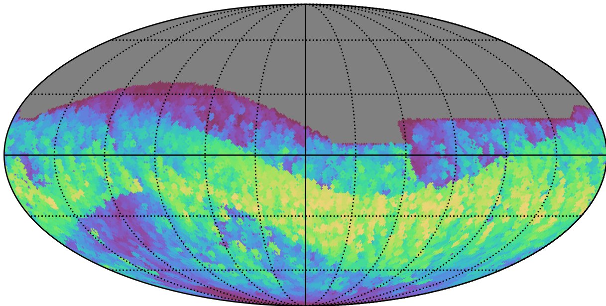
roman_v3.3_10yrs All sky i band: Max normairmass
