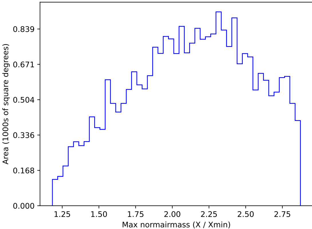
roman_v3.3_10yrs All sky i band: Max normairmass
