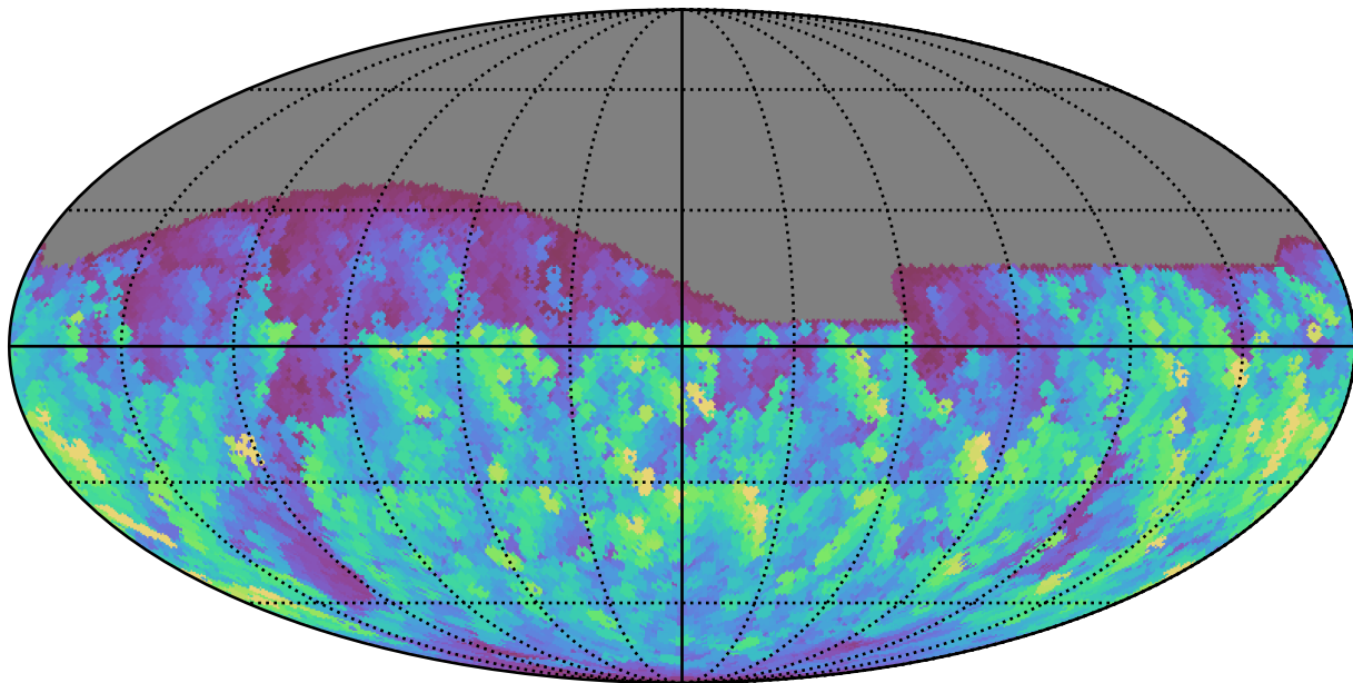
roman_v3.3_10yrs All sky g band: Max normairmass
