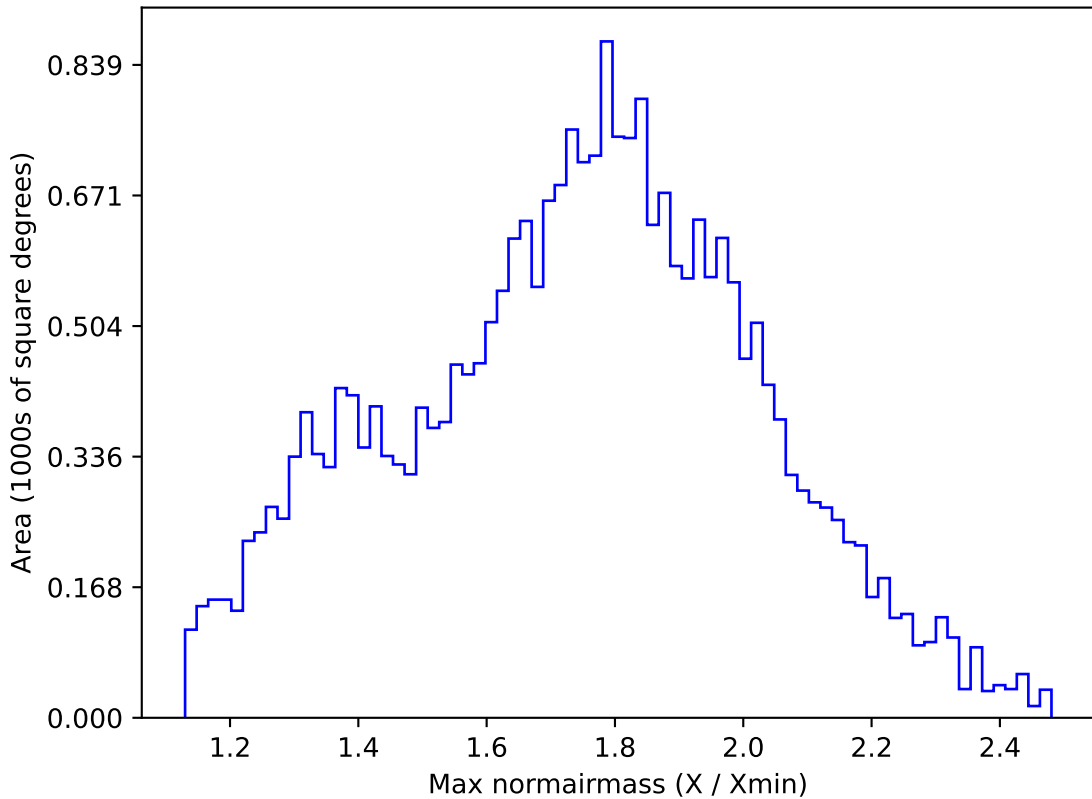
roman_v3.3_10yrs All sky g band: Max normairmass
