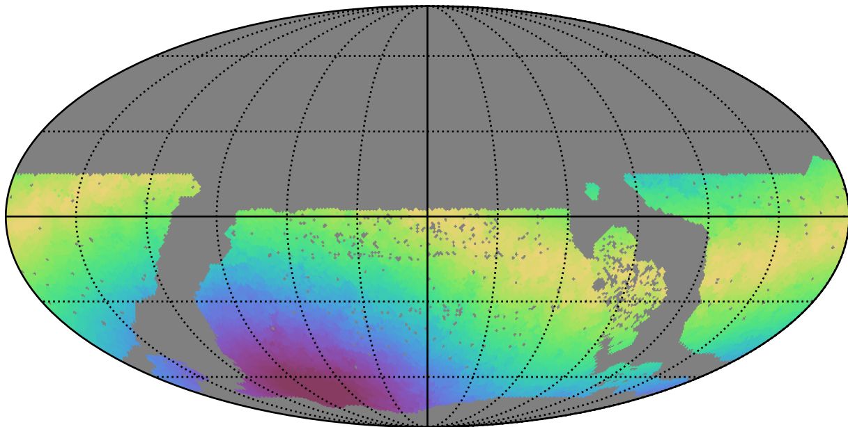
roman_v3.3_10yrs WFD z band: Max moonDistance
