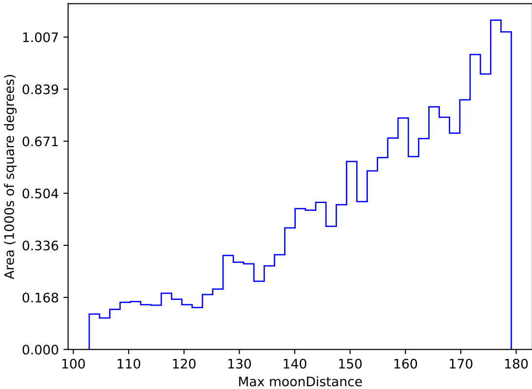
roman_v3.3_10yrs WFD z band: Max moonDistance
