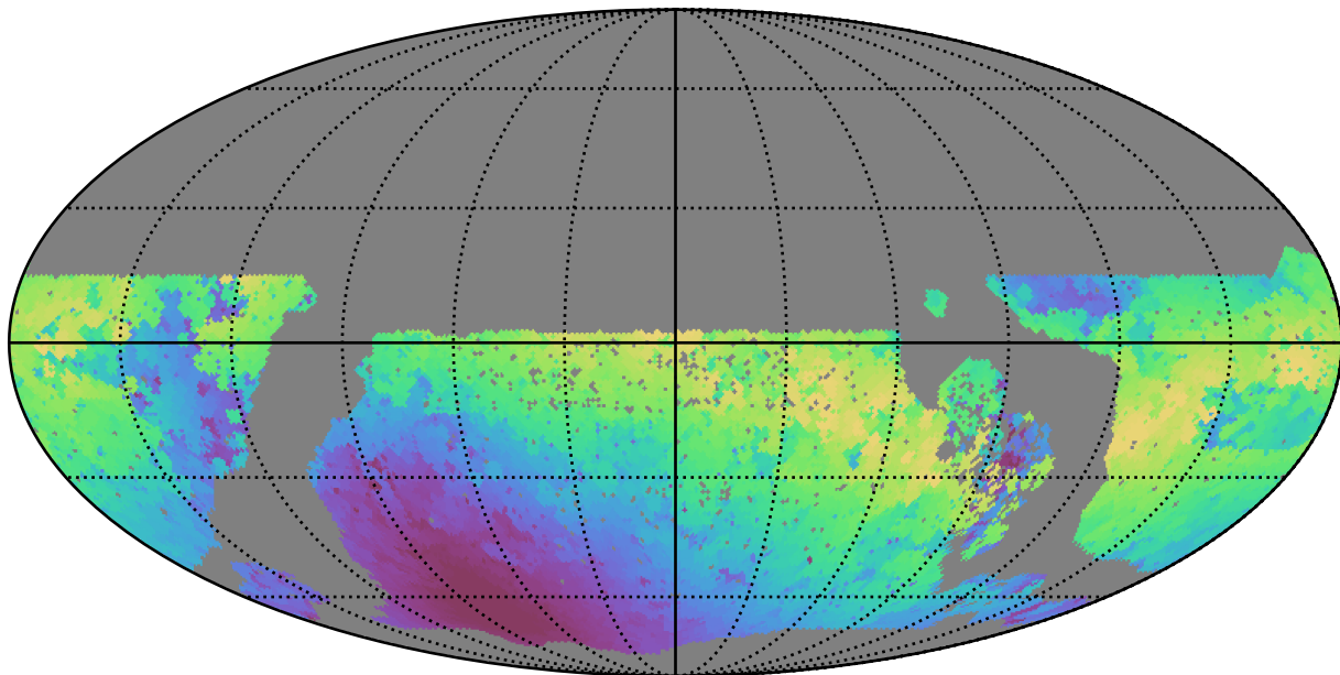
roman_v3.3_10yrs WFD y band: Max moonDistance
