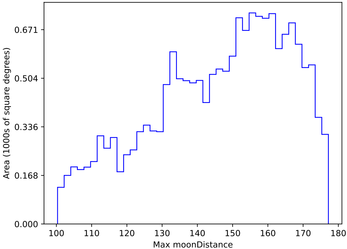
roman_v3.3_10yrs WFD y band: Max moonDistance
