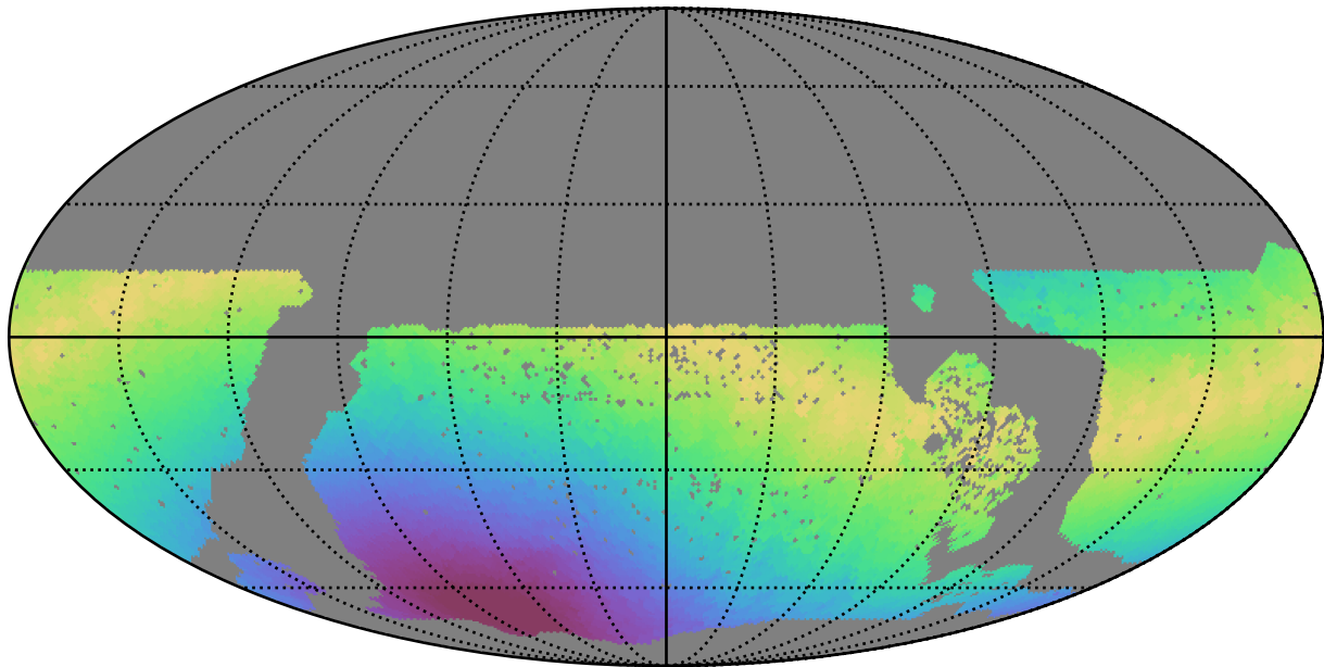
roman_v3.3_10yrs WFD u band: Max moonDistance
