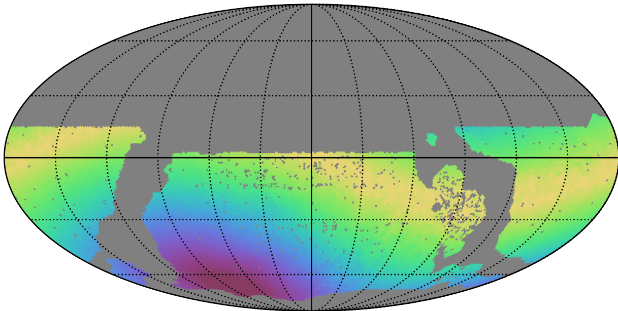
roman_v3.3_10yrs WFD r band: Max moonDistance
