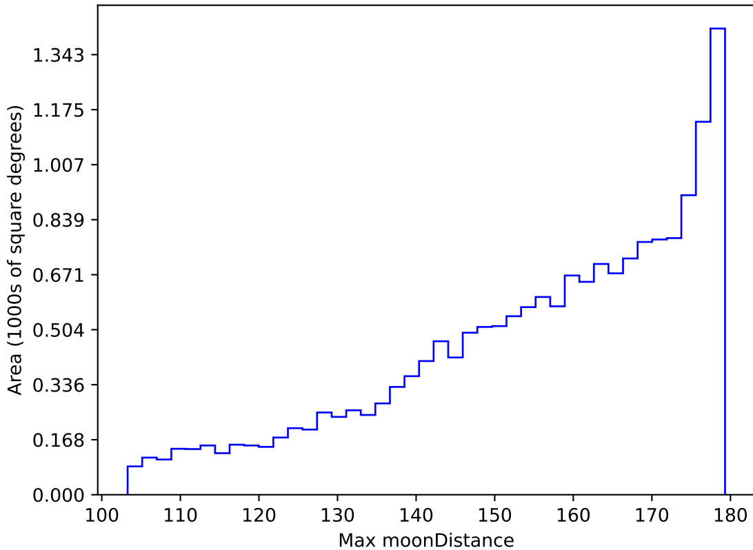
roman_v3.3_10yrs WFD r band: Max moonDistance
