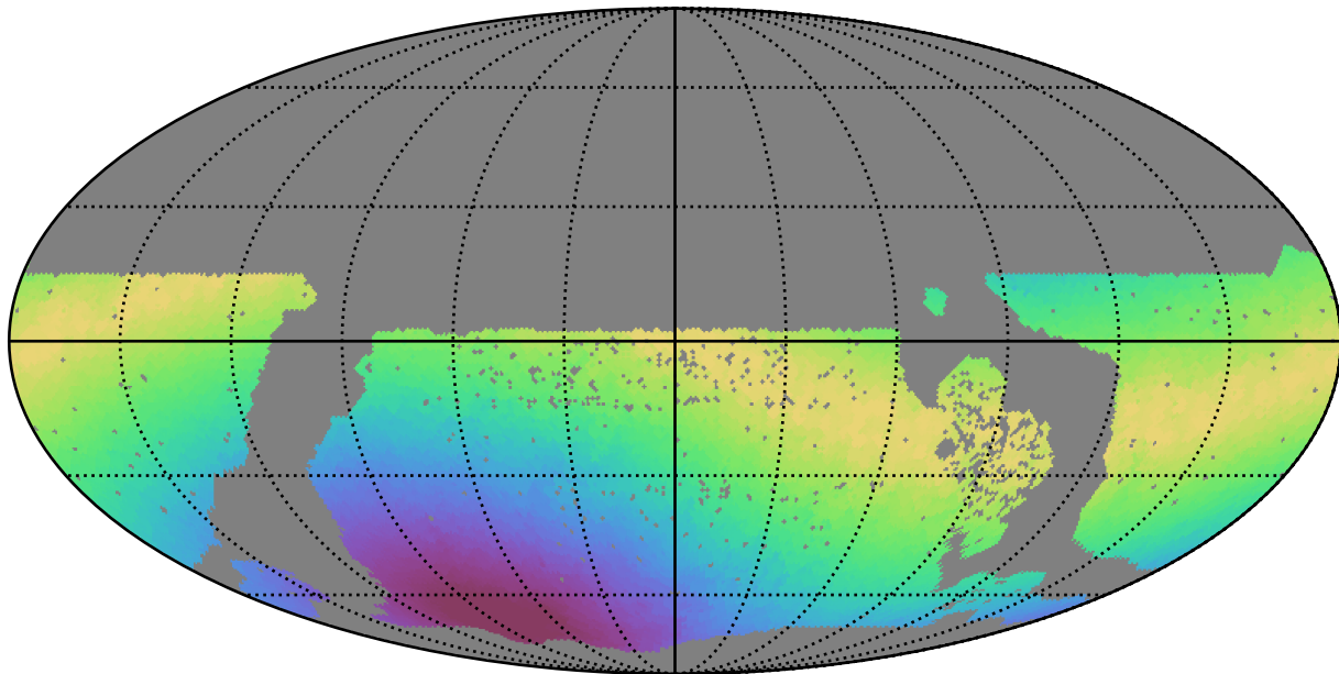
roman_v3.3_10yrs WFD i band: Max moonDistance
