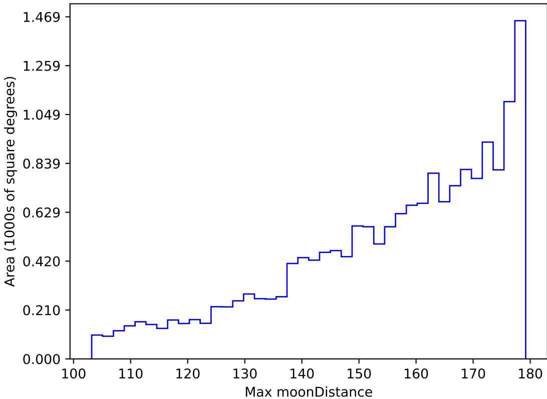
roman_v3.3_10yrs WFD i band: Max moonDistance
