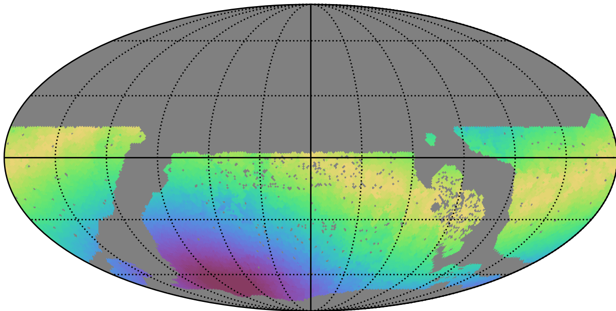
roman_v3.3_10yrs WFD g band: Max moonDistance
