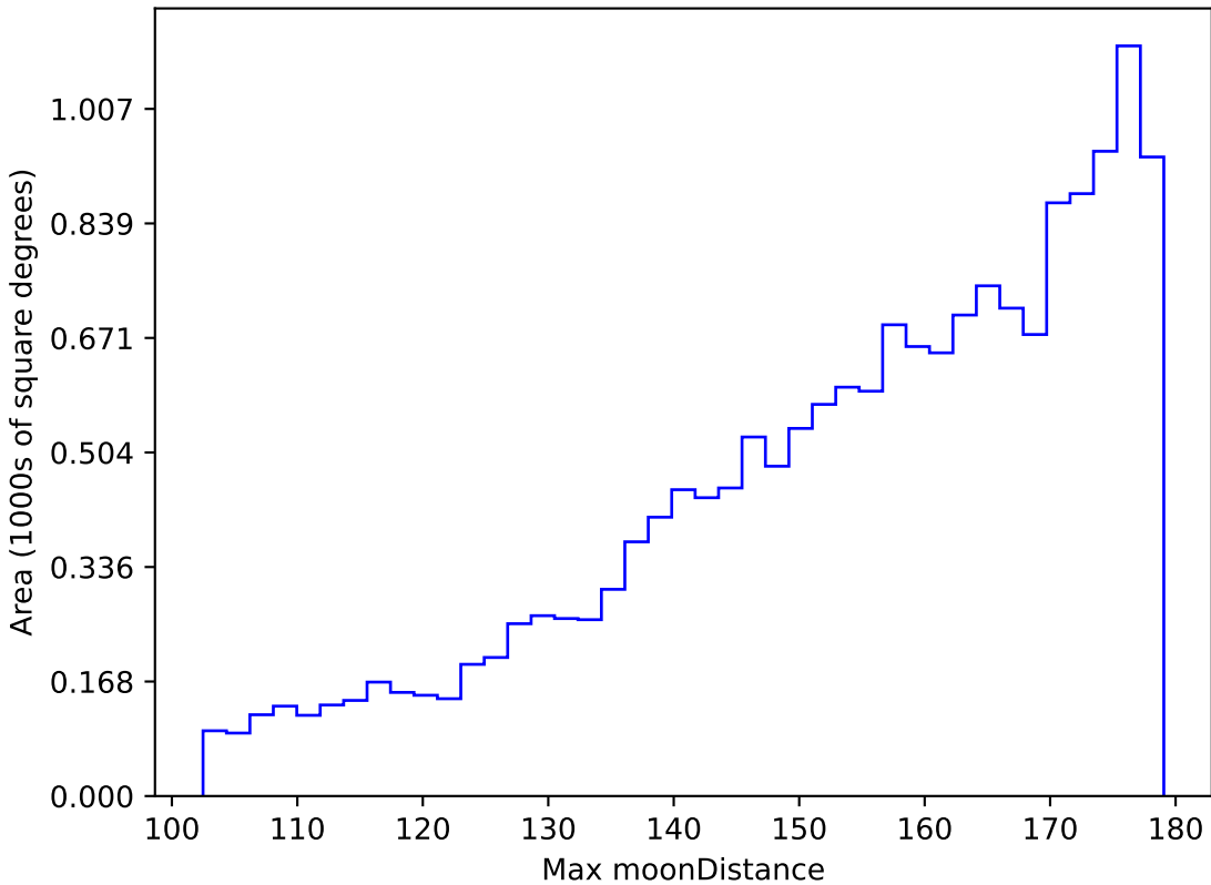
roman_v3.3_10yrs WFD g band: Max moonDistance
