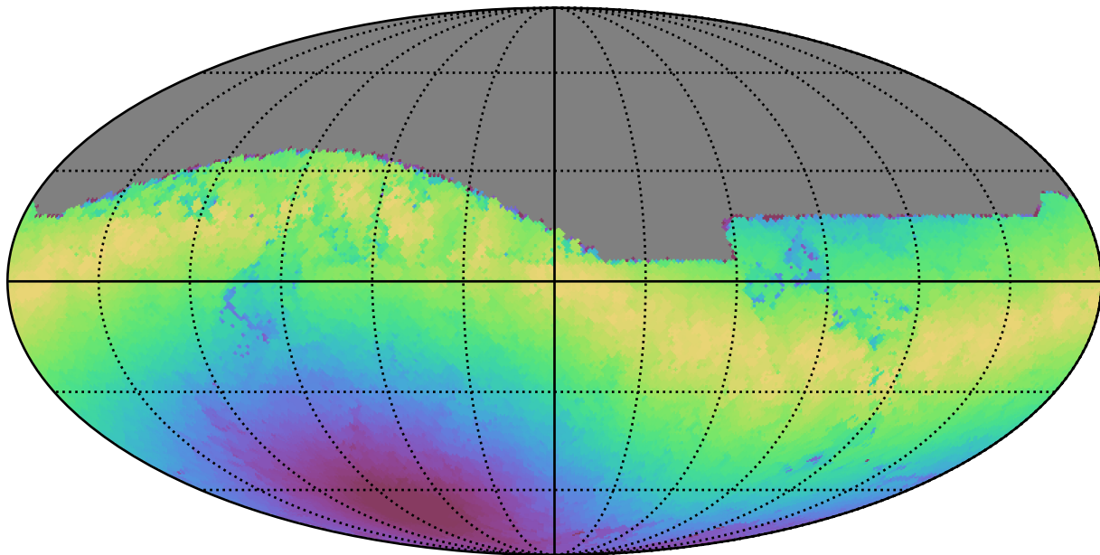
roman_v3.3_10yrs All sky z band: Max moonDistance
