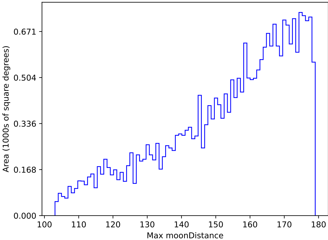
roman_v3.3_10yrs All sky z band: Max moonDistance
