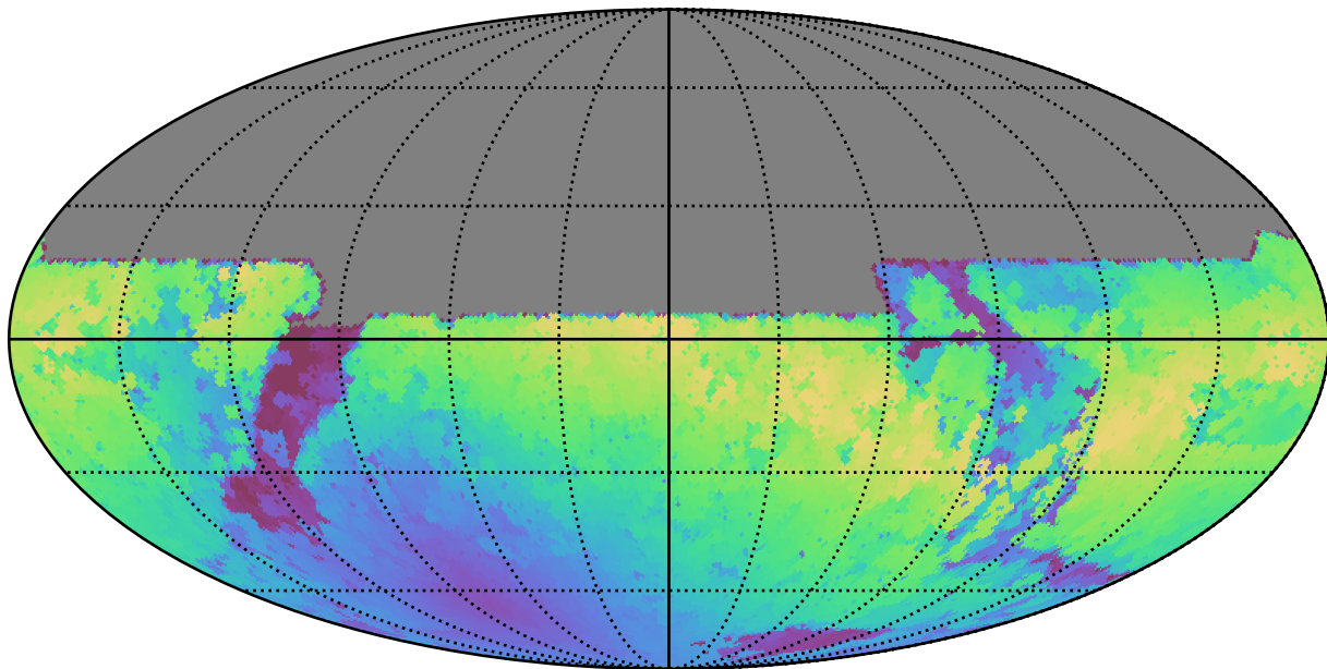
roman_v3.3_10yrs All sky y band: Max moonDistance
