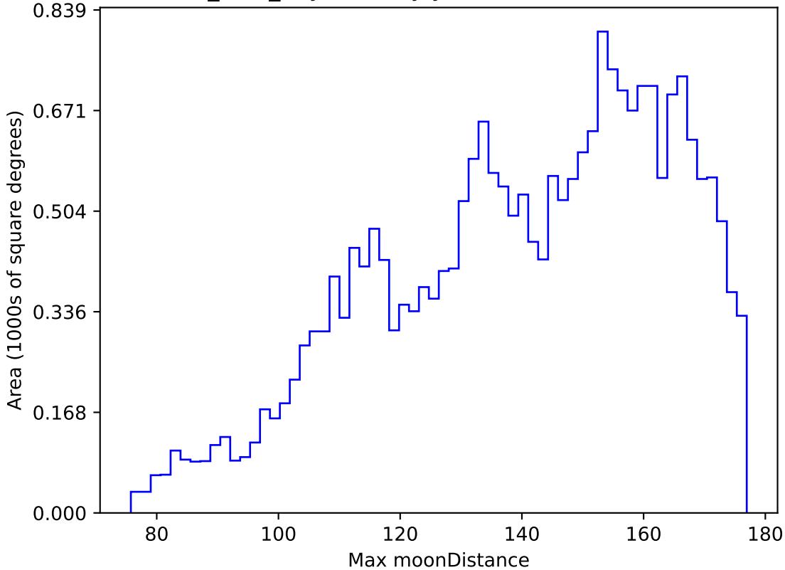
roman_v3.3_10yrs All sky y band: Max moonDistance
