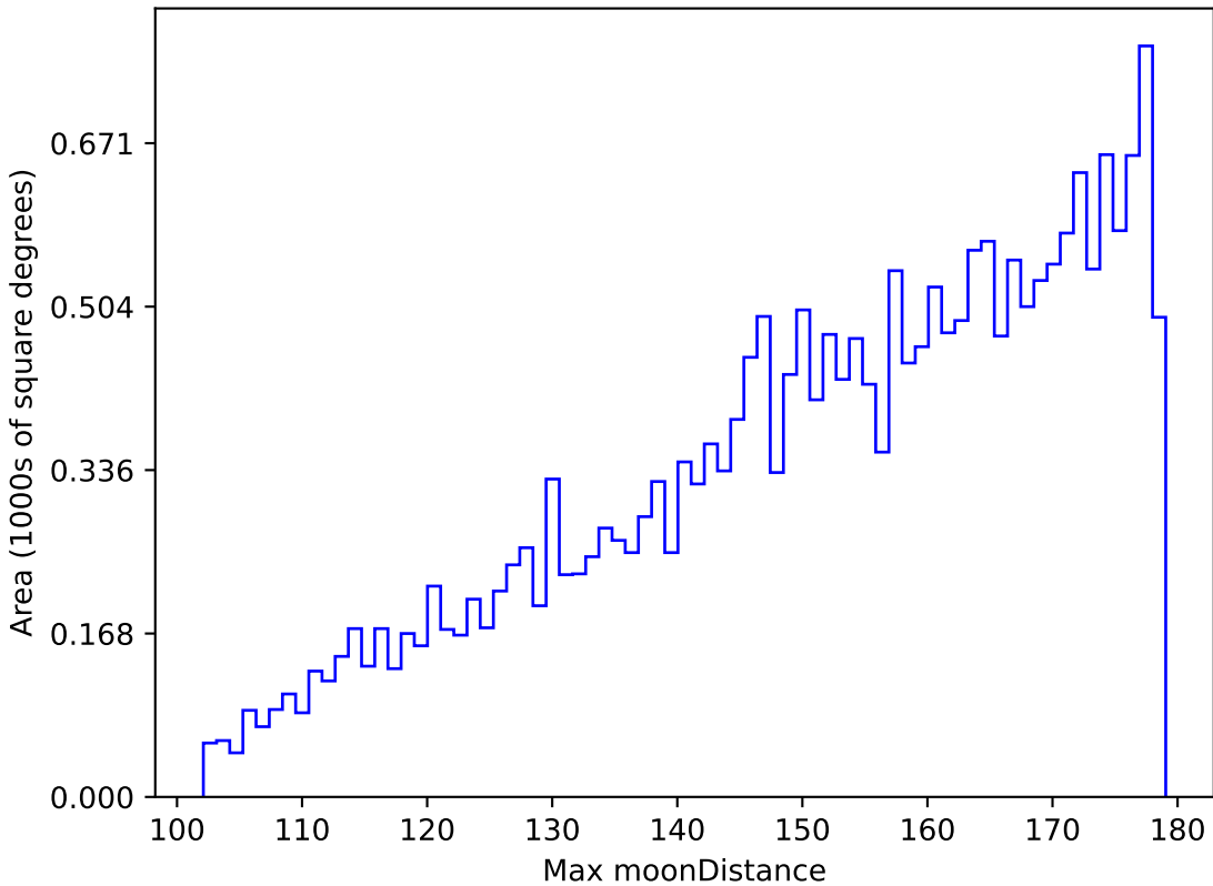
roman_v3.3_10yrs All sky u band: Max moonDistance
