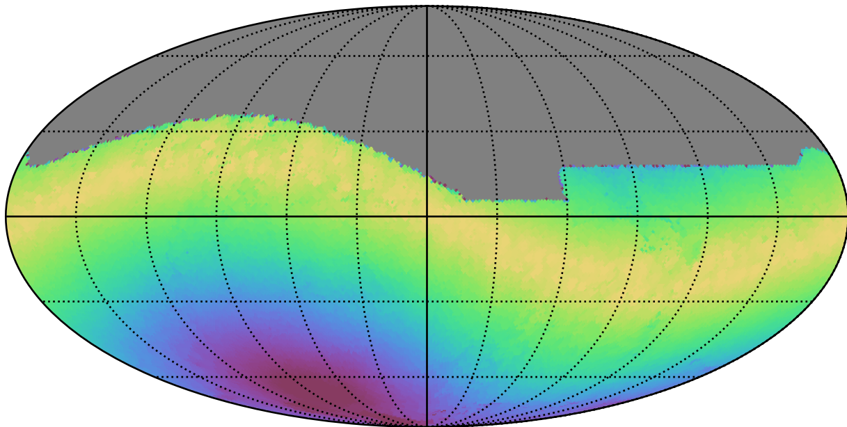
roman_v3.3_10yrs All sky r band: Max moonDistance
