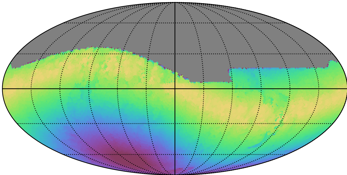
roman_v3.3_10yrs All sky i band: Max moonDistance
