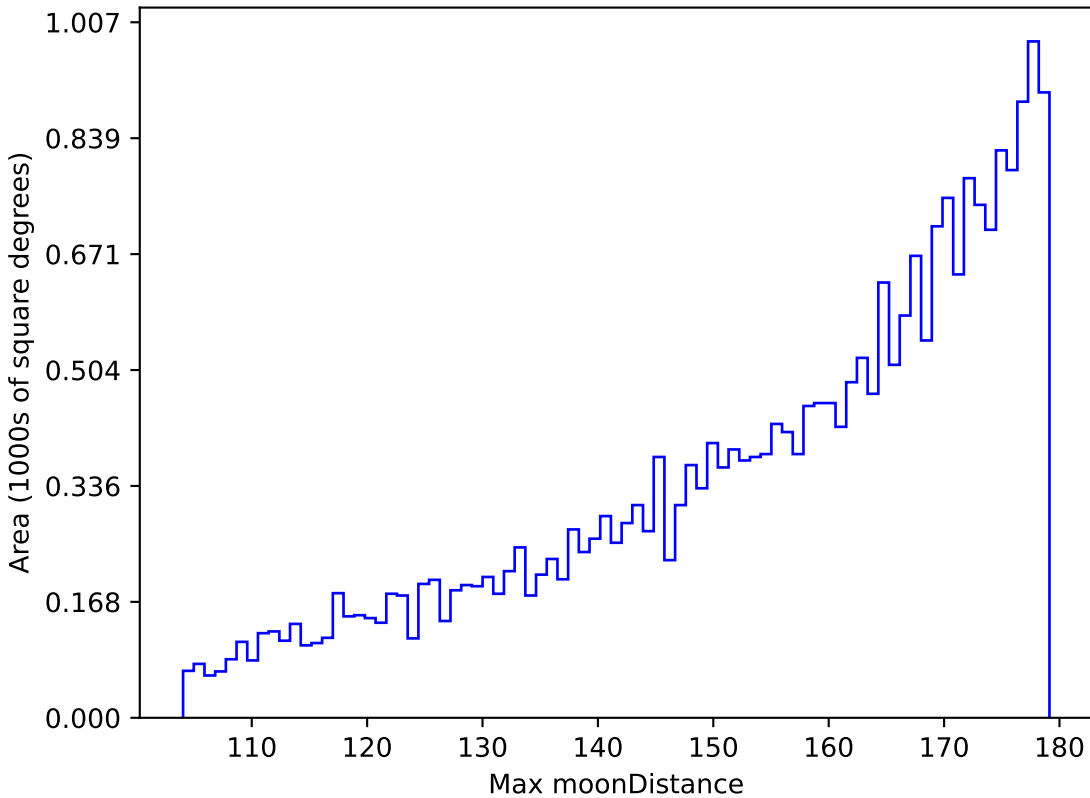
roman_v3.3_10yrs All sky i band: Max moonDistance
