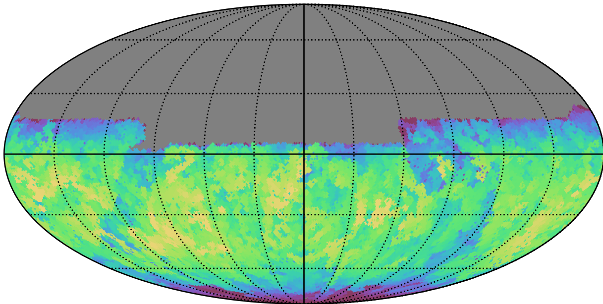
roman_v3.3_10yrs Yr 1 y band: Max fiveSigmaDepth
