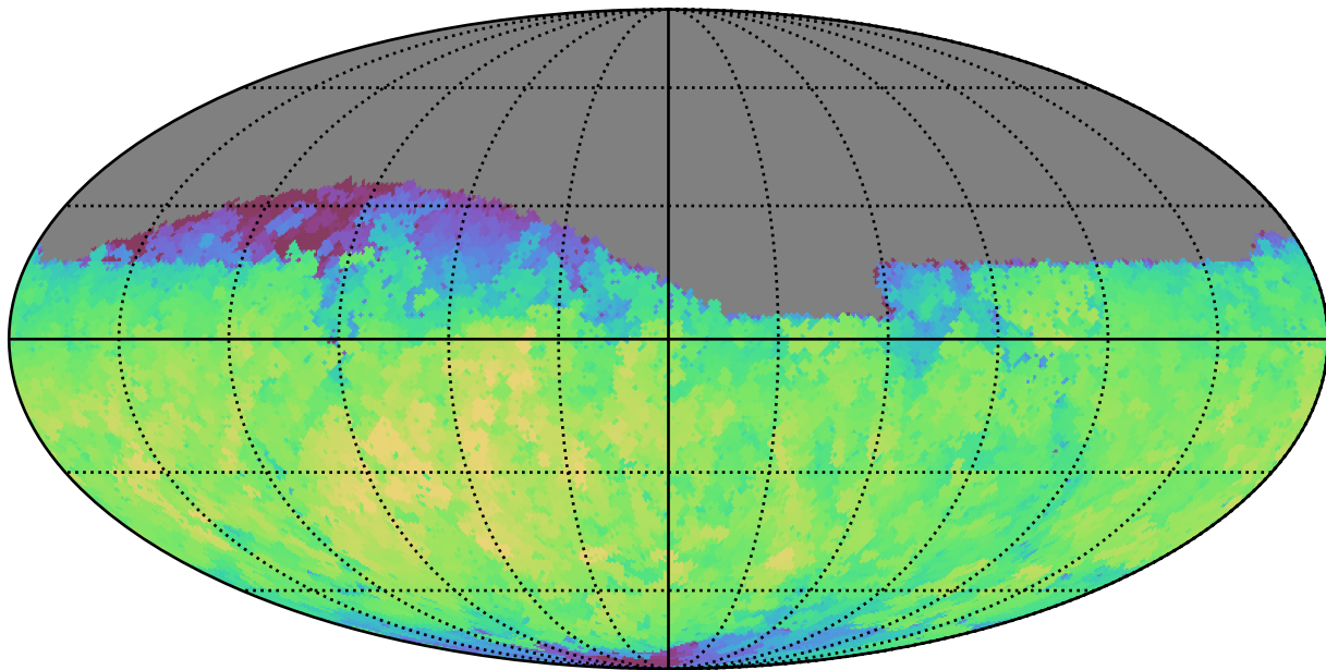
roman_v3.3_10yrs Yr 1 i band: Max fiveSigmaDepth
