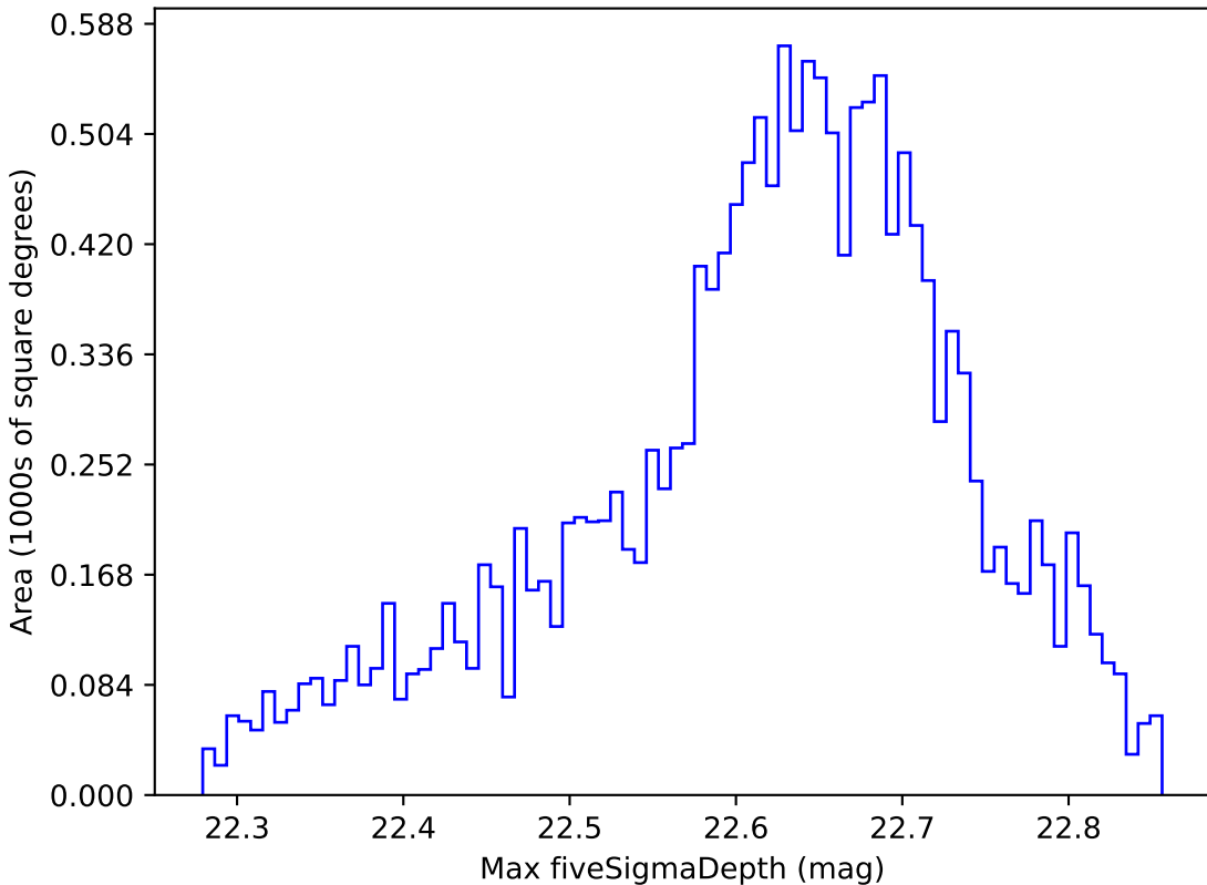
roman_v3.3_10yrs WFD y band: Max fiveSigmaDepth
