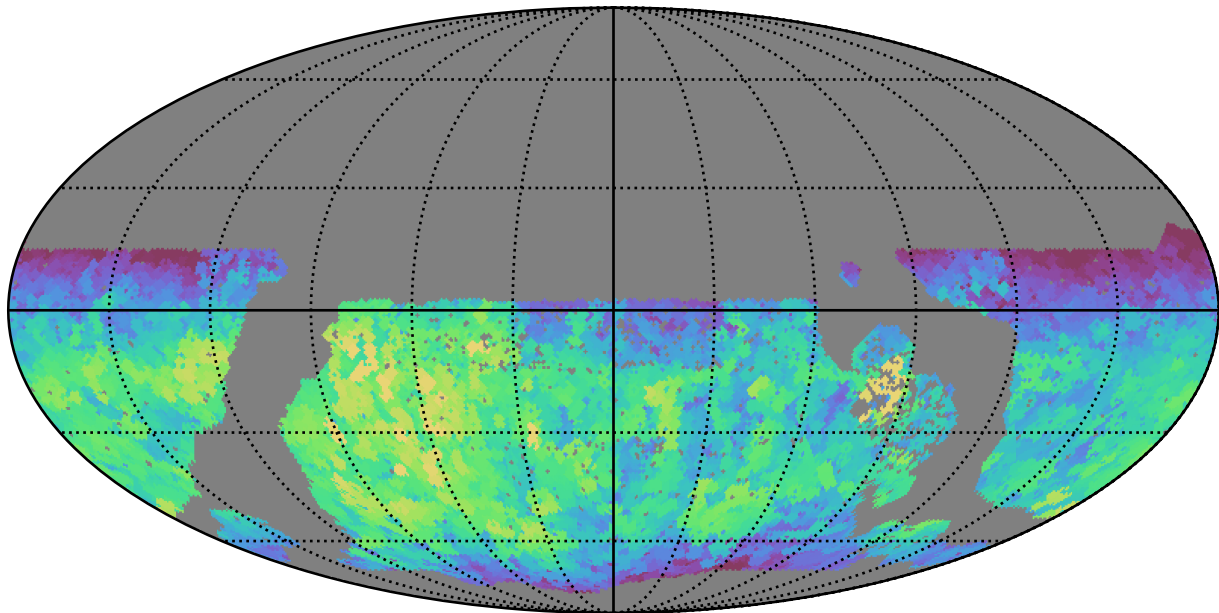
roman_v3.3_10yrs WFD i band: Max fiveSigmaDepth
