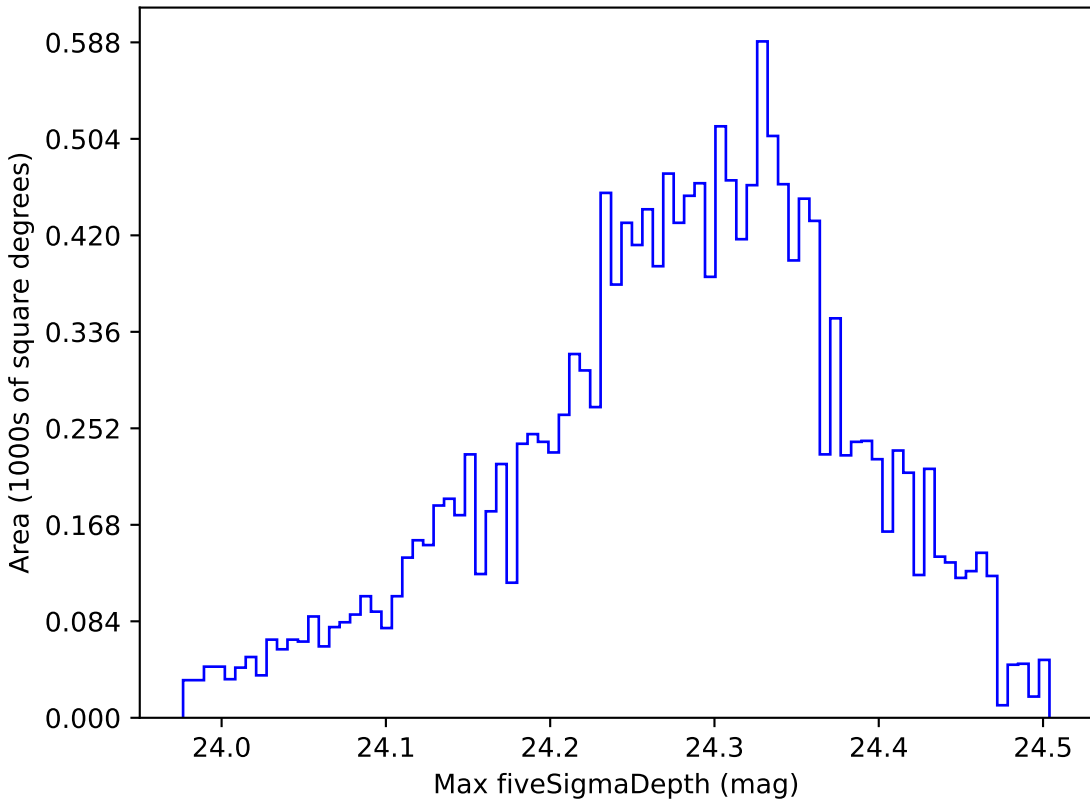
roman_v3.3_10yrs WFD i band: Max fiveSigmaDepth
