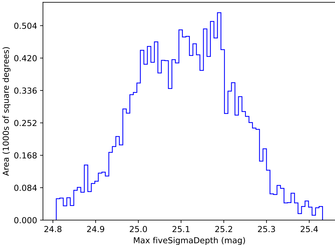
roman_v3.3_10yrs WFD g band: Max fiveSigmaDepth
