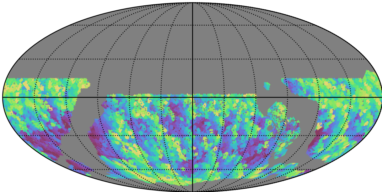
roman_v3.3_10yrs WFD y band: Max airmass
