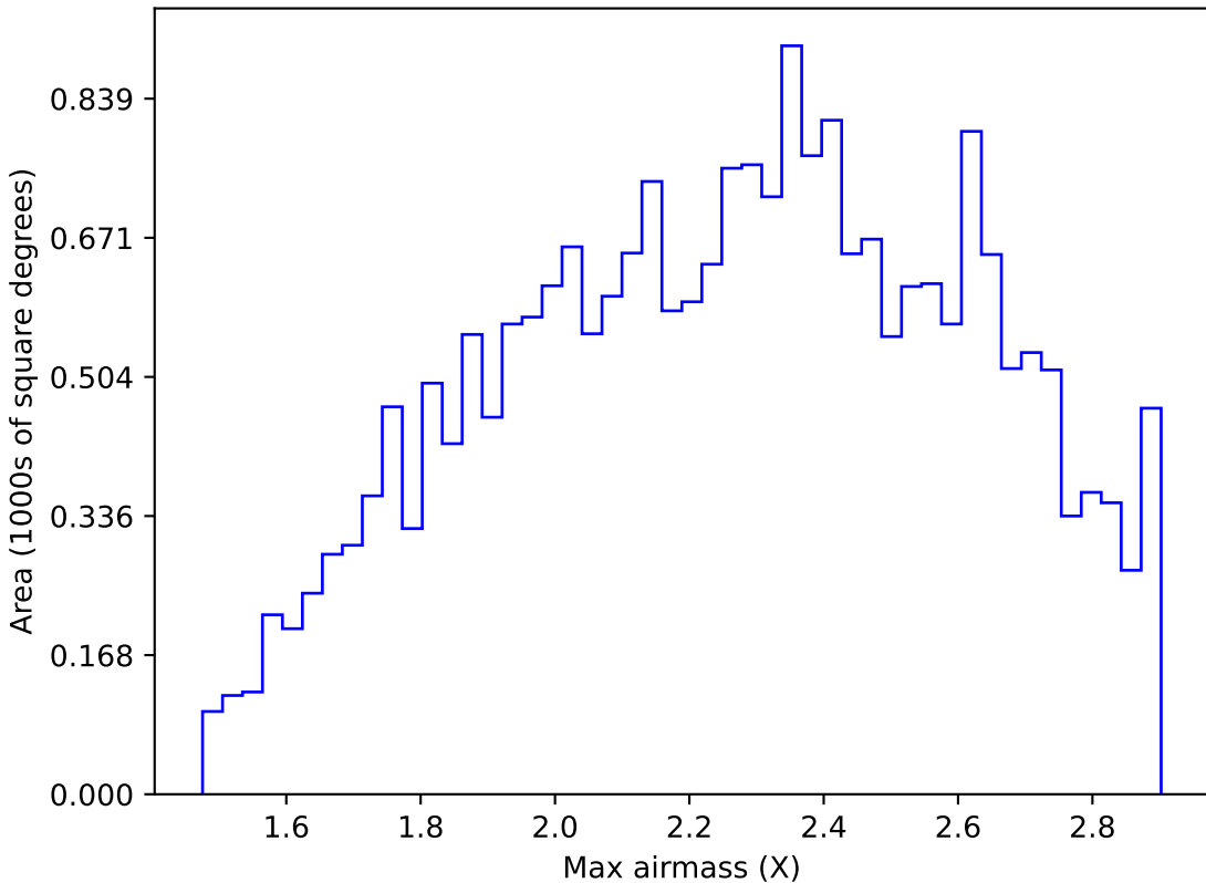
roman_v3.3_10yrs All sky y band: Max airmass
