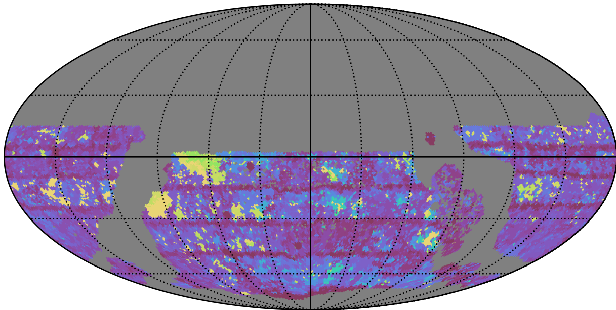
roman_v3.3_10yrs WFD y band: Max Inter-Night Gap
