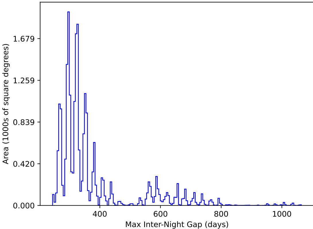
roman_v3.3_10yrs All sky y band: Max Inter-Night Gap
