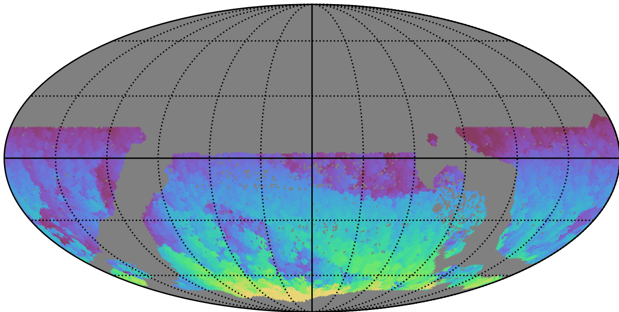
roman_v3.3_10yrs WFD z band: Max HA
