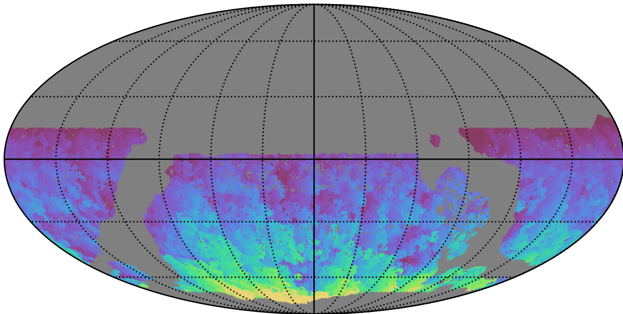
roman_v3.3_10yrs WFD y band: Max HA
